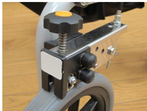
WA-0ブレーキ写真
